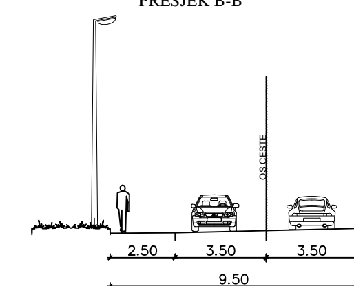
PRESJEK B-B
