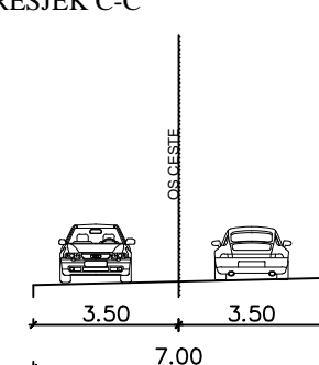
PRESJEK C-C
